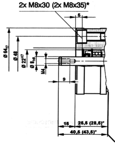
編碼器驅動裝置 Q
