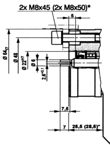
轉速表驅動裝置 T
