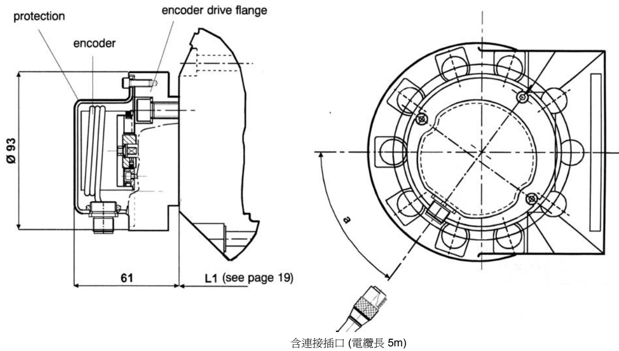
增量型編碼器
