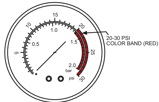
Indicator Gauge (25 PSI)
