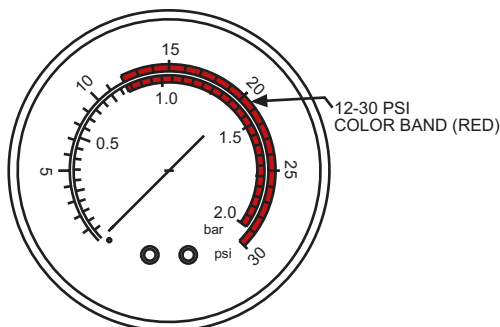
Indicator Gauge (15 PSI)
