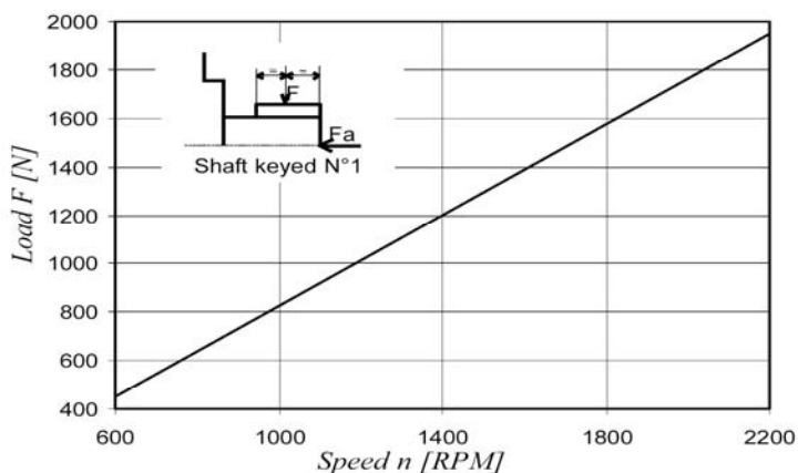
PERMISSIBLE RADIAL LOAD
