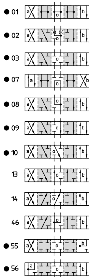
閥芯位置 04 先導閥帶 2 定位機構
