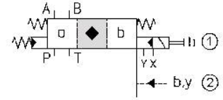
閥芯位置 05 彈簧對中
