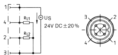
插座接線圖
