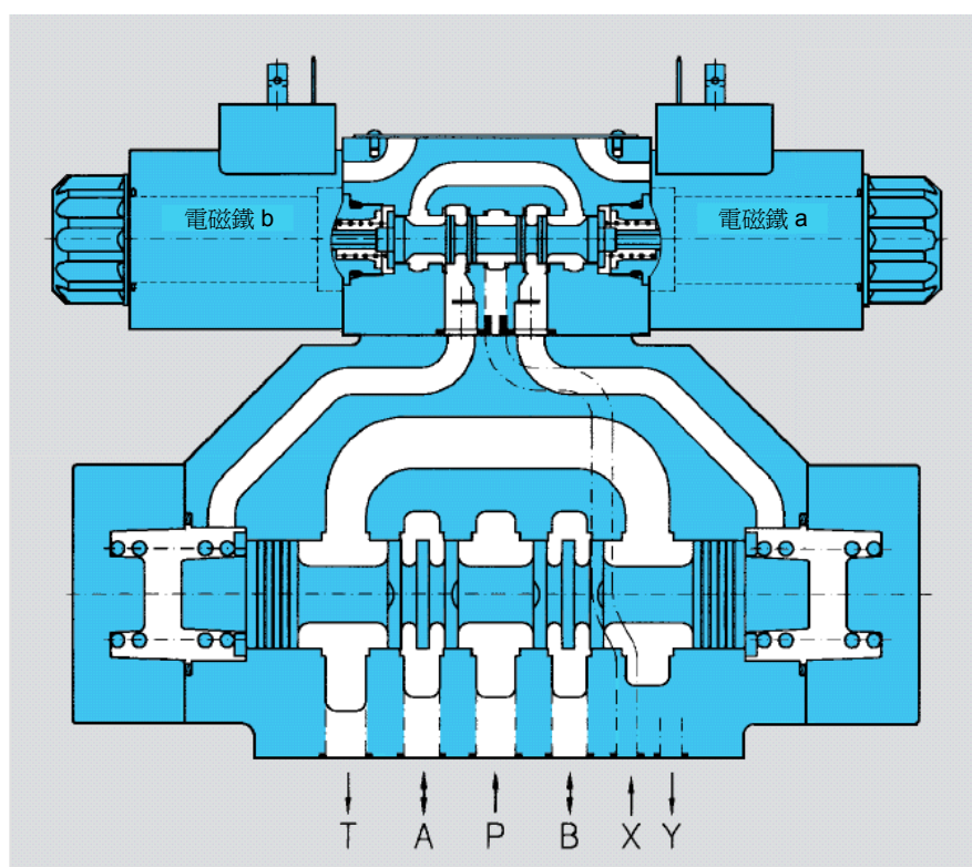
結構簡圖（圖示為 DC 電液方向閥）
