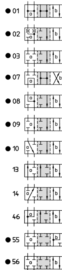
閥芯位置 02 彈簧偏置
