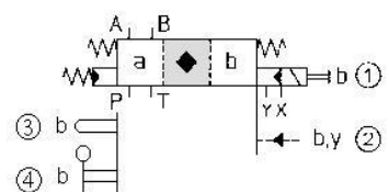
閥芯位置 02 彈簧偏置
