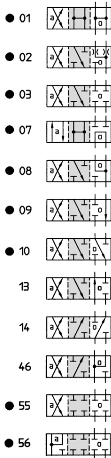
閥芯位置 01 彈簧偏置
