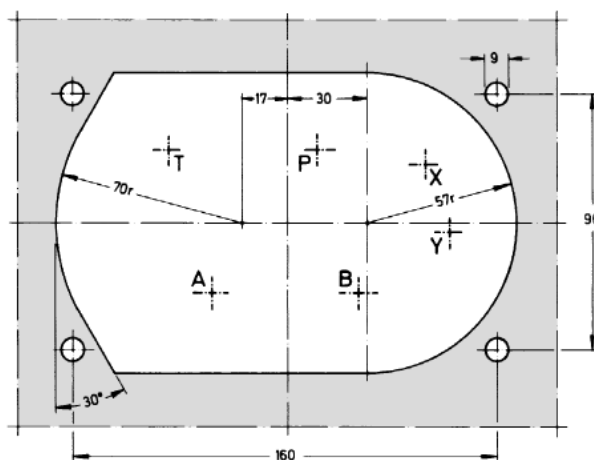
面板開孔尺寸（適用於 G1" 安裝底板）
